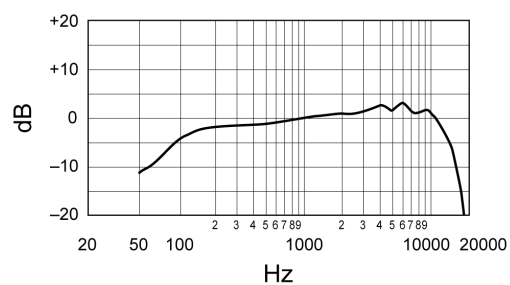
Typischer Frequenzgang
